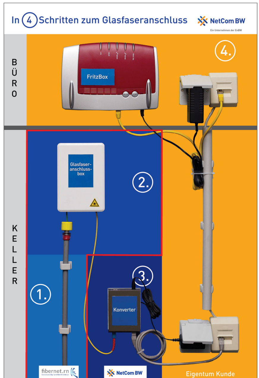
Schematische Darstellung der Glasfaseranschluss-Komponenten
