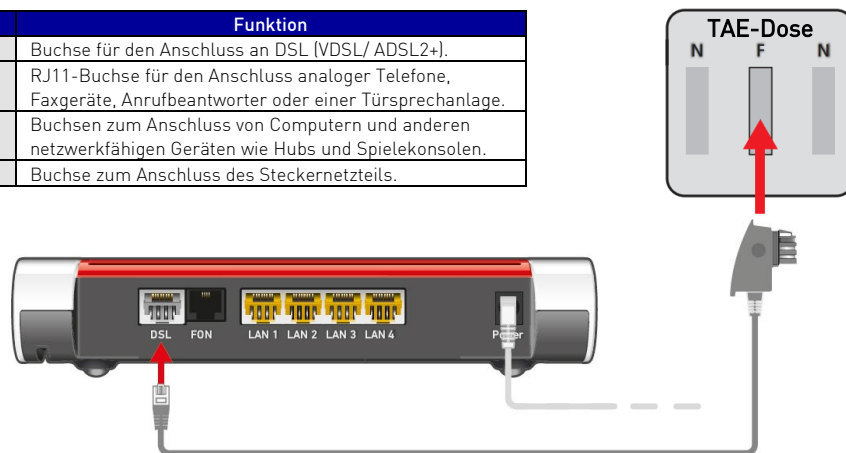
Verbindung mit dem DSL-Anschluss herstellen
